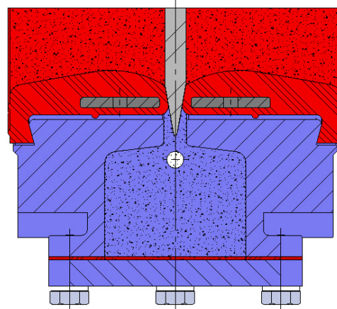
SECTION D-D
